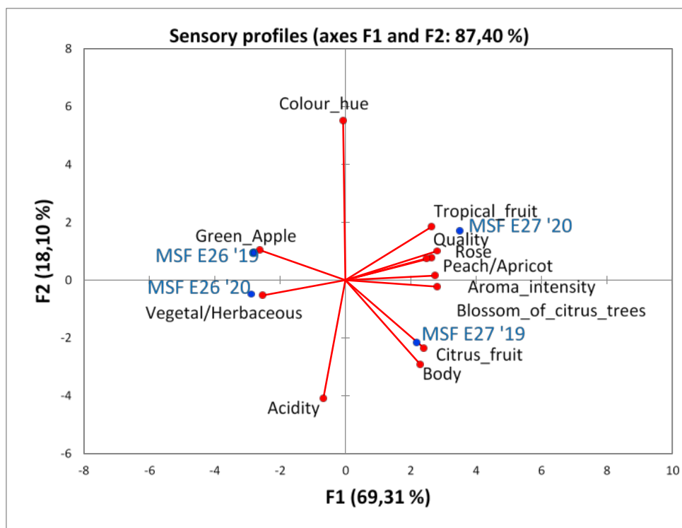
Διάγραμμα PCA (Principal Component Analysis) από την οργανοληπτική αξιολόγηση των δύο κλώνων Μοσχοφίλερο των τρύγων 2019 και 2020 όπου απεικονίζονται τα δείγματα οίνων (μπλε κουκίδες) και οι περιγραφικοί όροι (κόκκινα διανύσματα)
